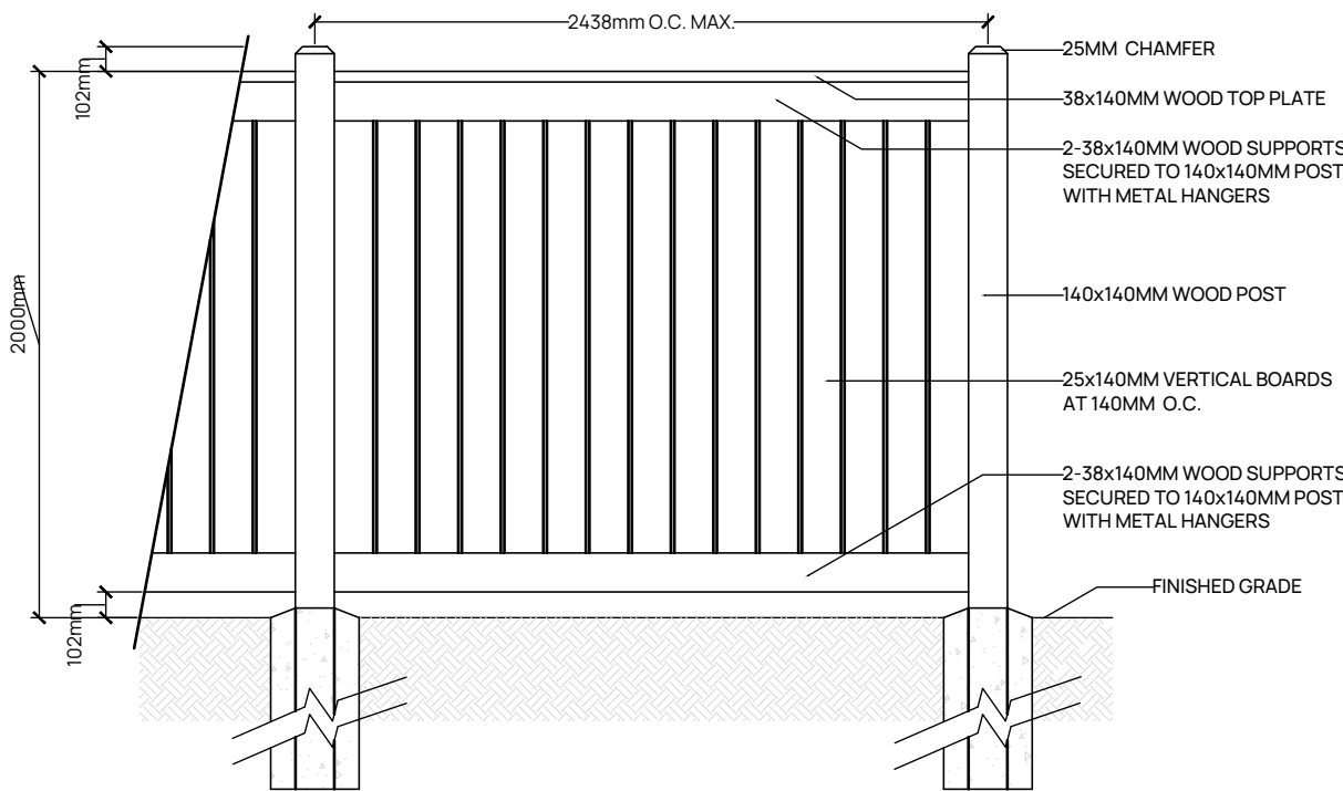
ELEVATION
