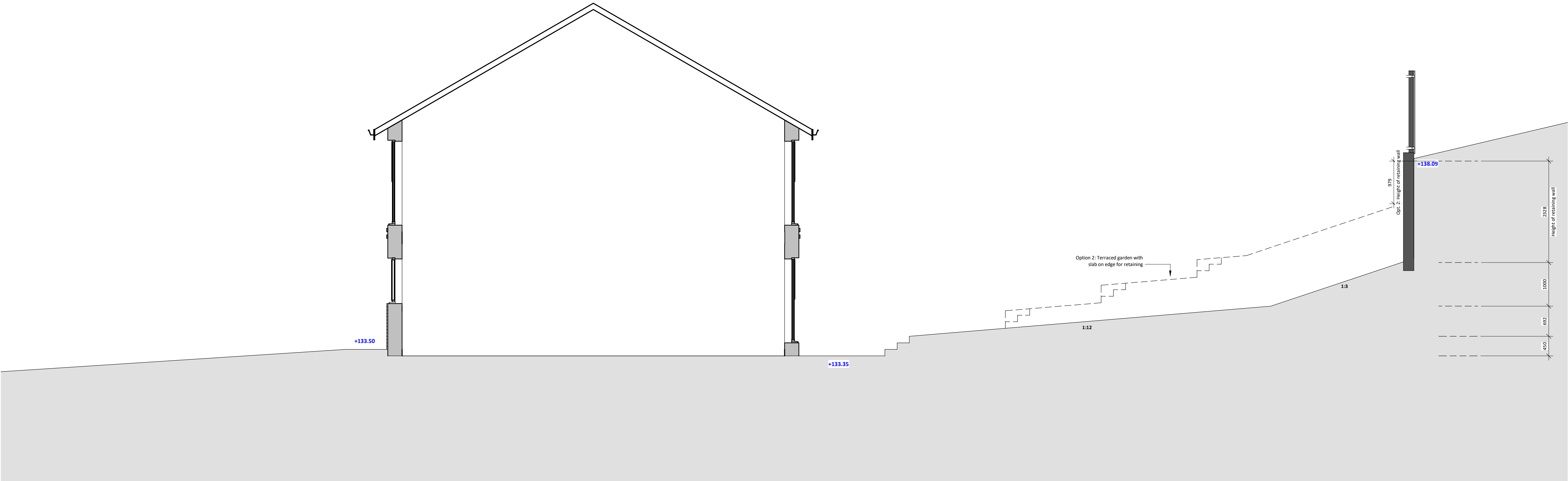
Plot 15 Section 1 : 50
