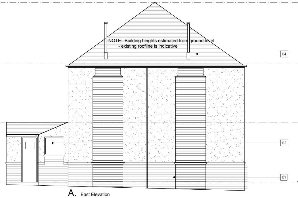
A. East Elevation
