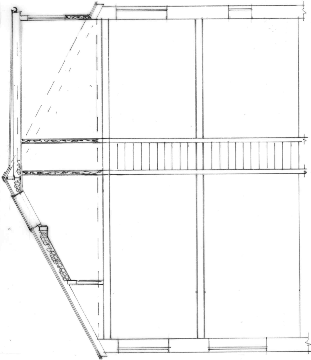
SECTION A.A
