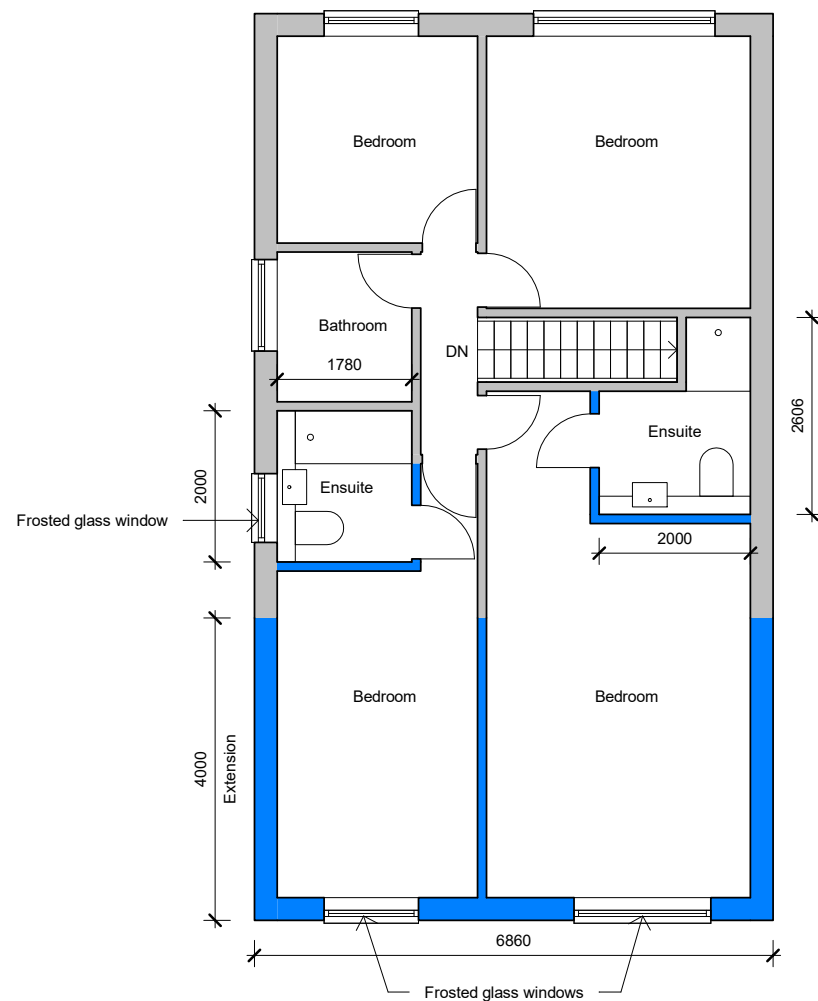
2 Level 1 1 : 100
