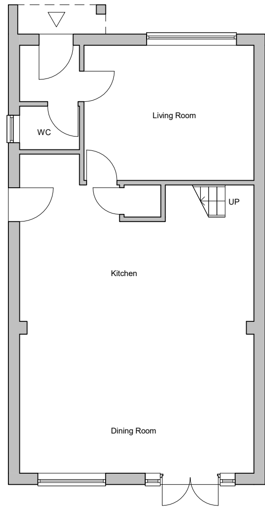
1 Level 0 1 : 100
