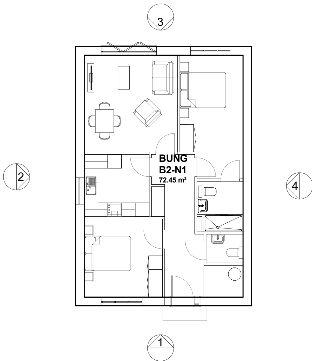
00_ BUNGALOW B2-N1 FLOOR PLAN 1 : 100
