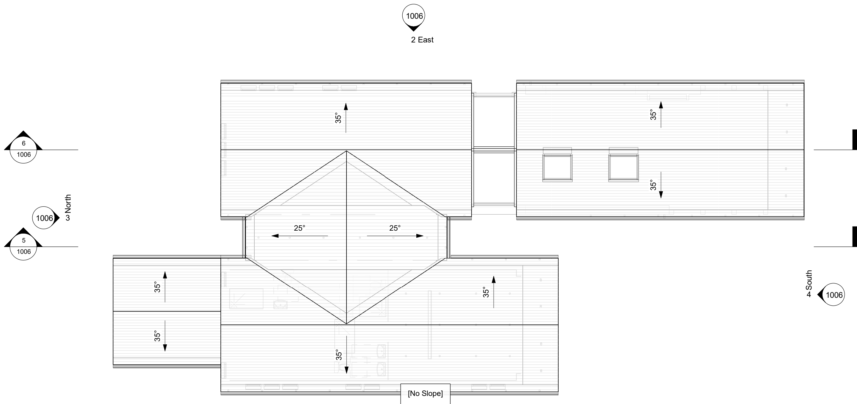
Roof Plan 1 : 100
