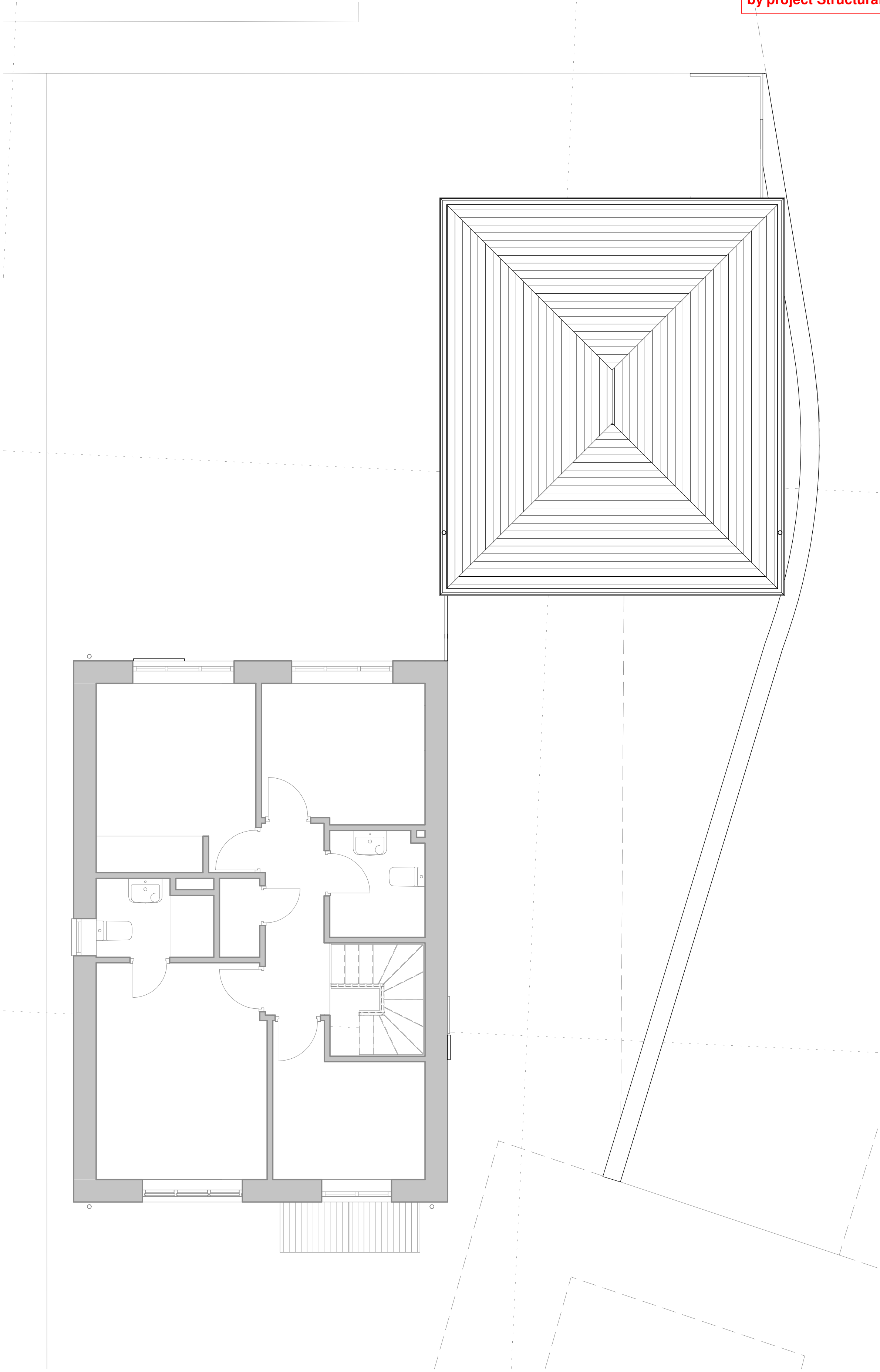
2 | Pro Roof Plan 1 : 50
