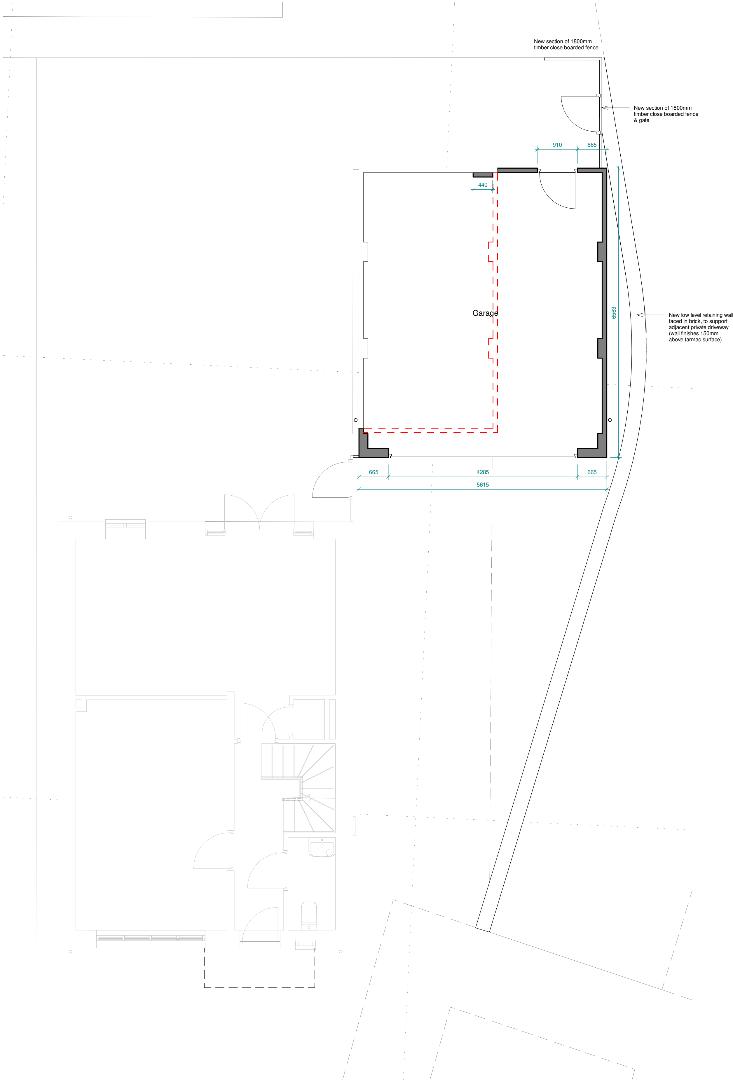
1 | Pro Level 0 1 : 50
