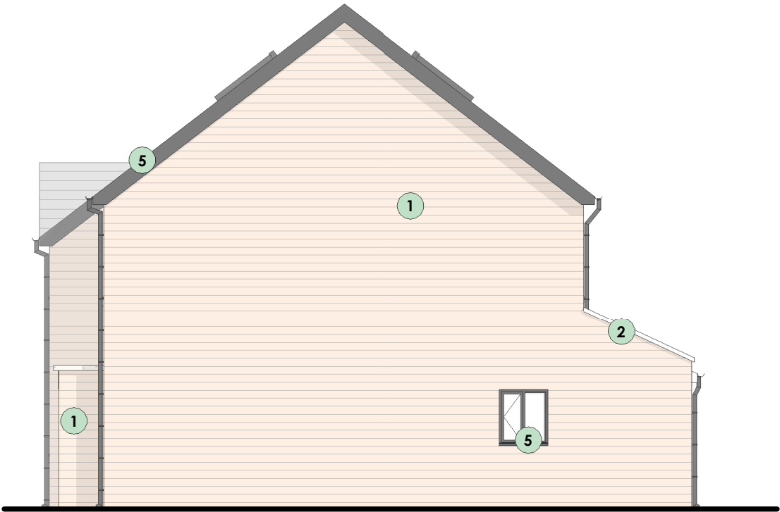
House Type A - Right (NMA) 1 : 100
