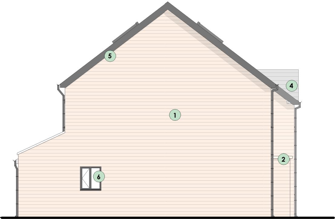
House Type A - Left (NMA) 1 : 100
