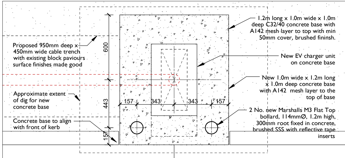
PLAN 1:20
