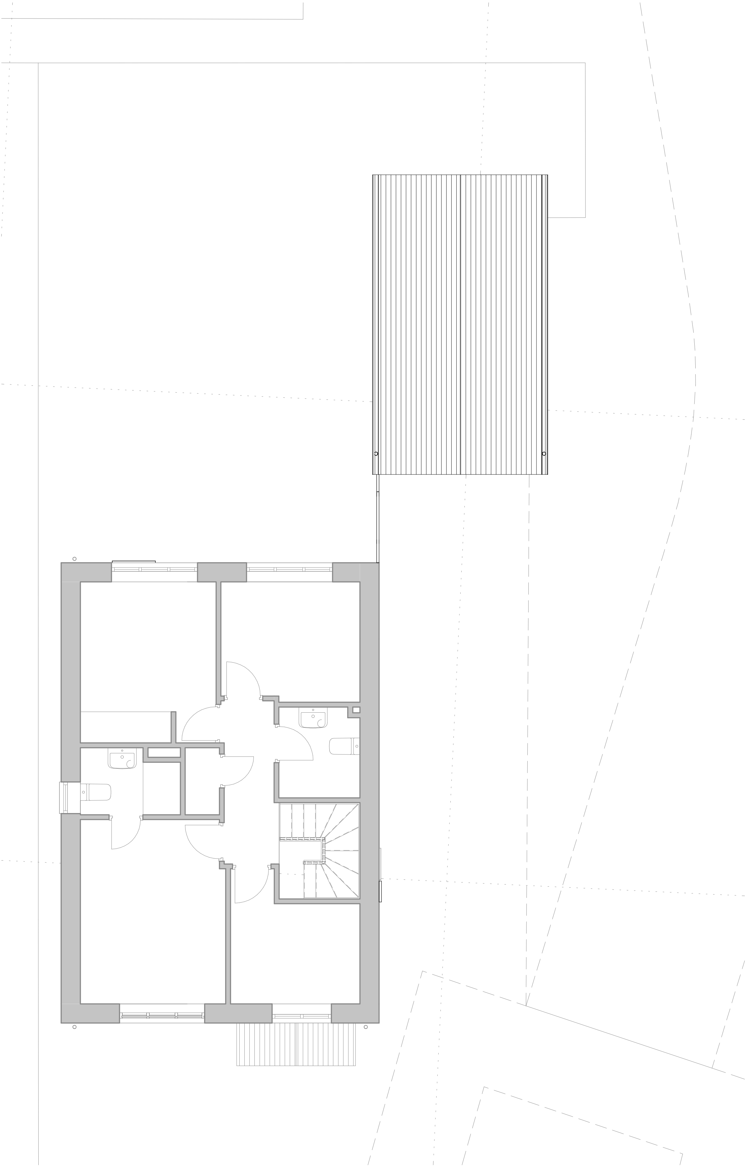
2 | Ex Roof Plan 1 : 50
