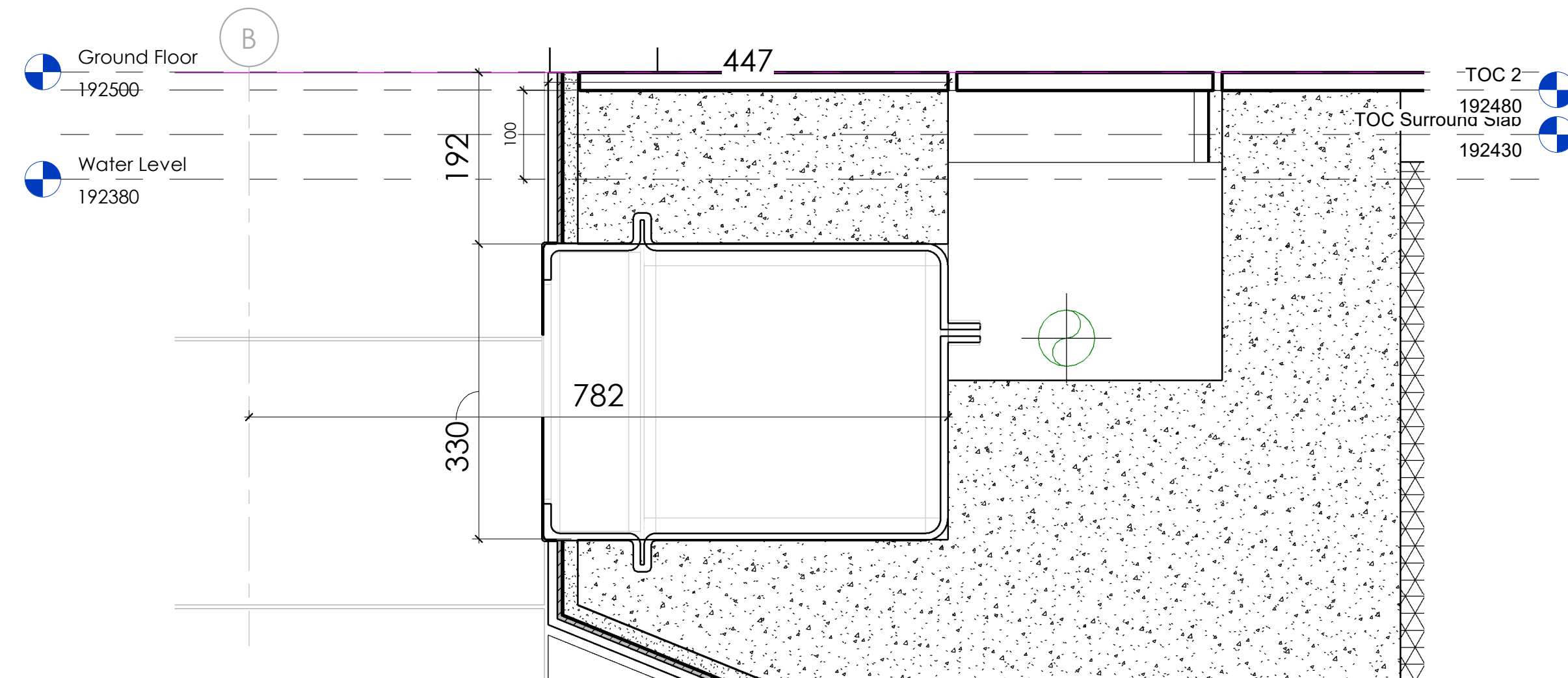
5 Eva Detail 1 : 5
