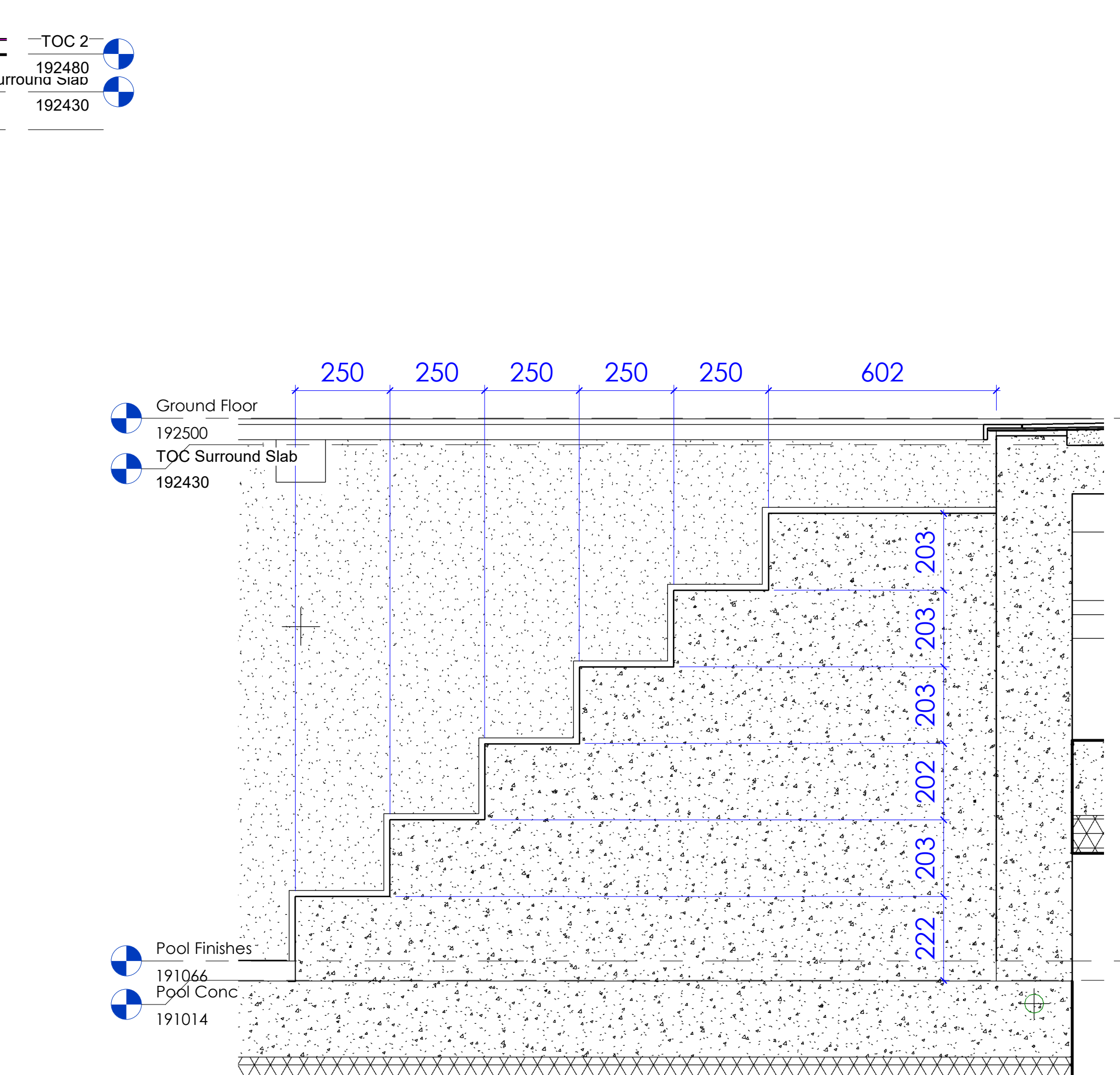
4 Conc Stairs 1 : 10
