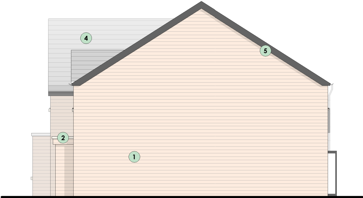
House Type B - Right (NMA) 1 : 100
