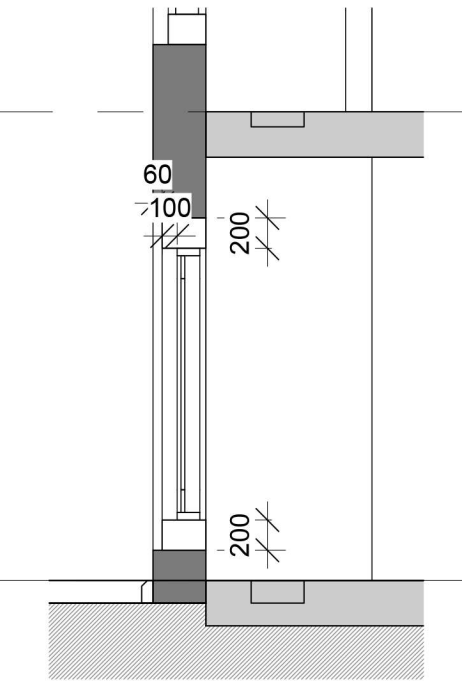
3 Section 2 1 : 50
