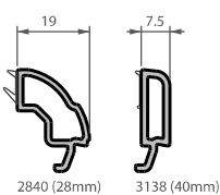
2840 (28mm)
