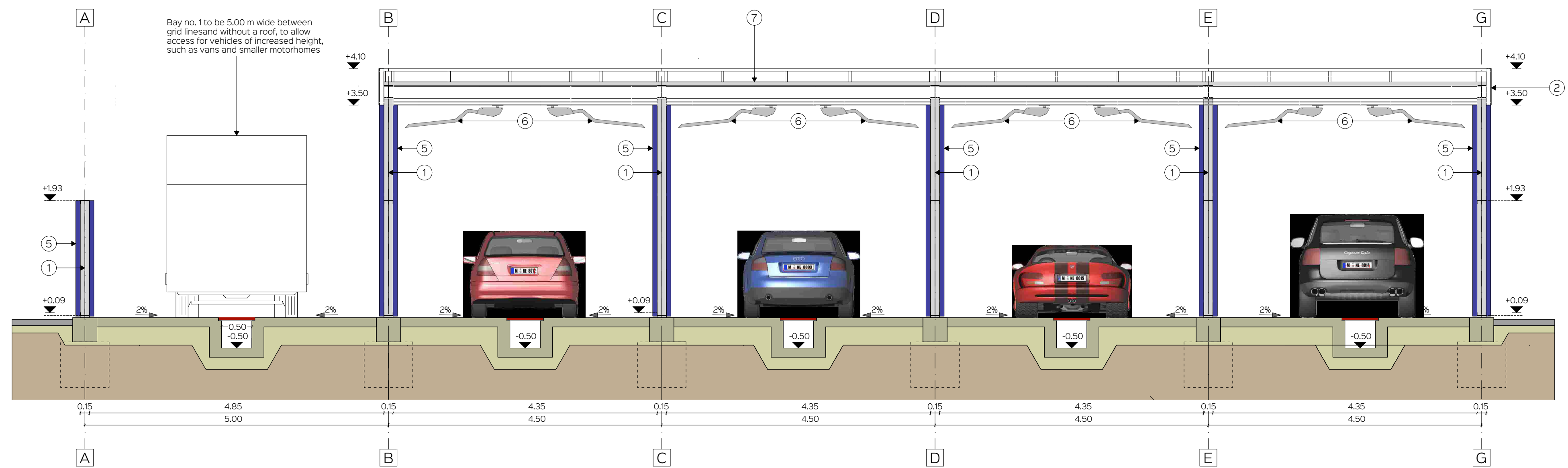
Long Section B - B (scale 1:50)
