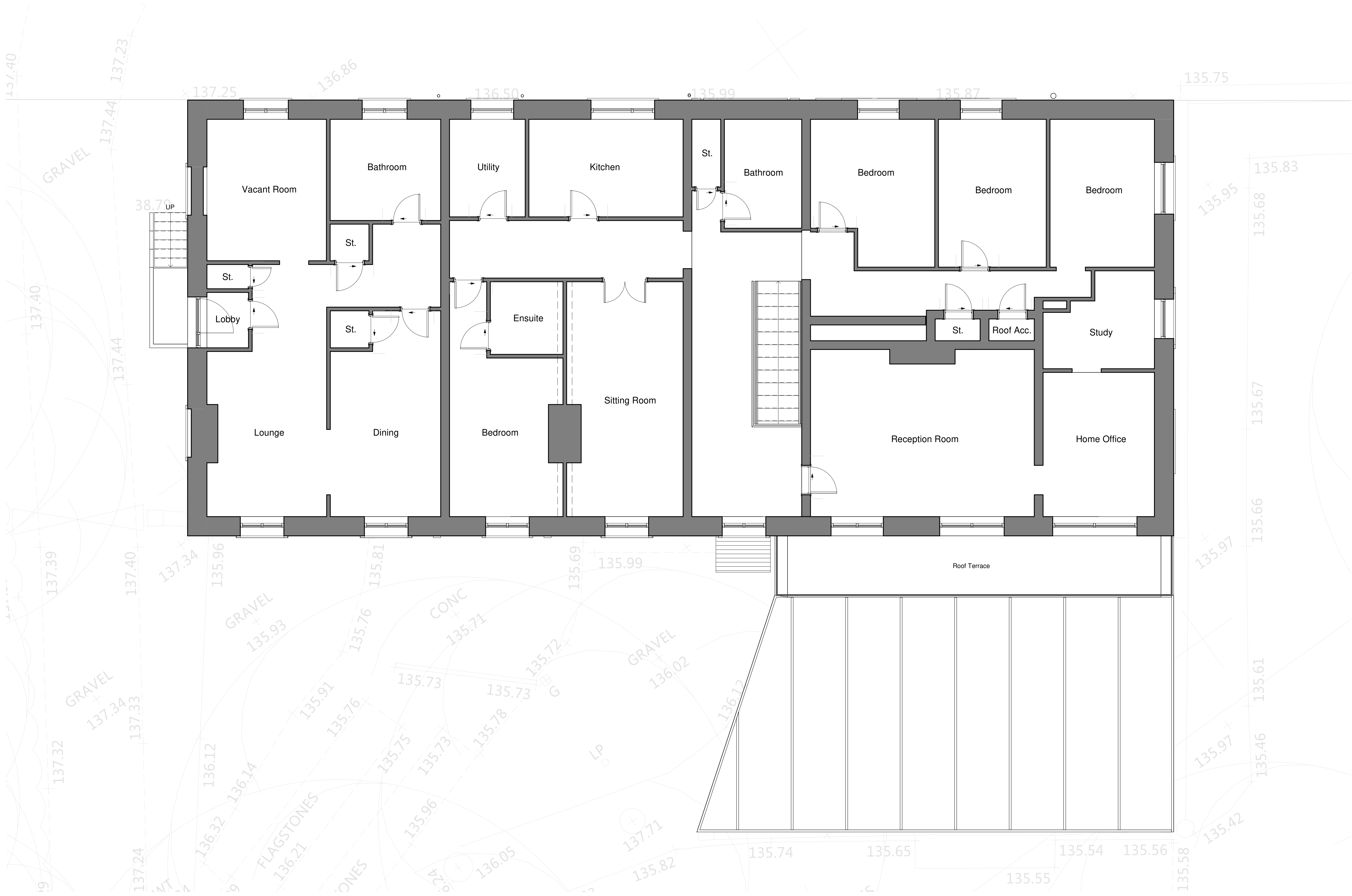
1 Existing Level 1 1 : 50
