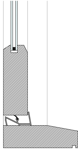
Sill: Inward Opening Door
