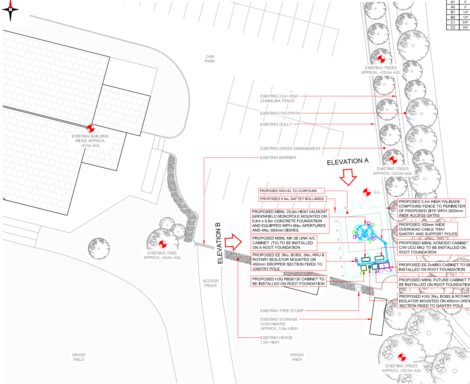
MAX CONFIGURATION SITE PLAN
