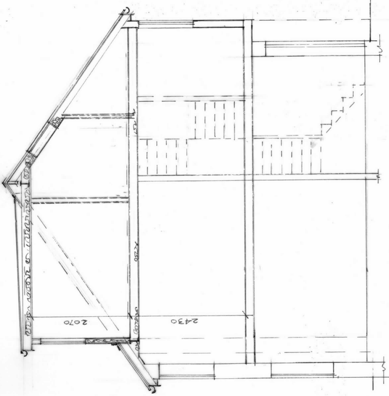
SECTION A.A
