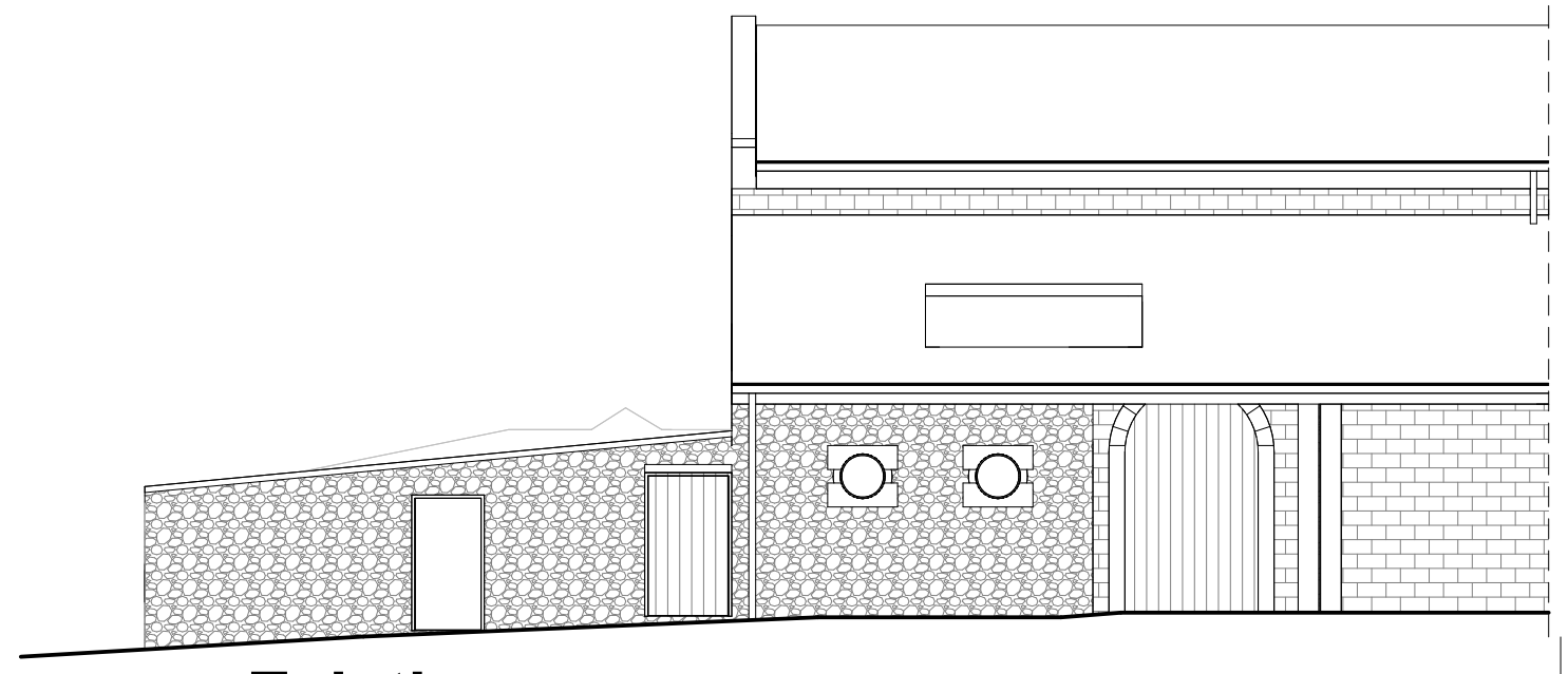
4 Existing 1 : 100
