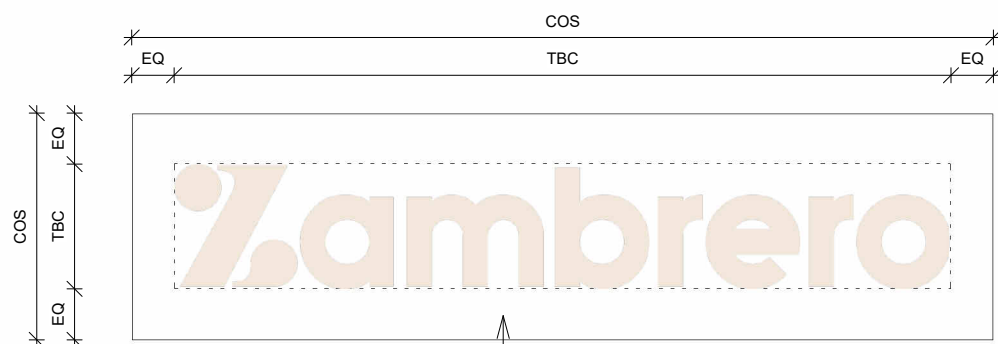
1 SIGN 03 - PYLON D200 1 : 10
