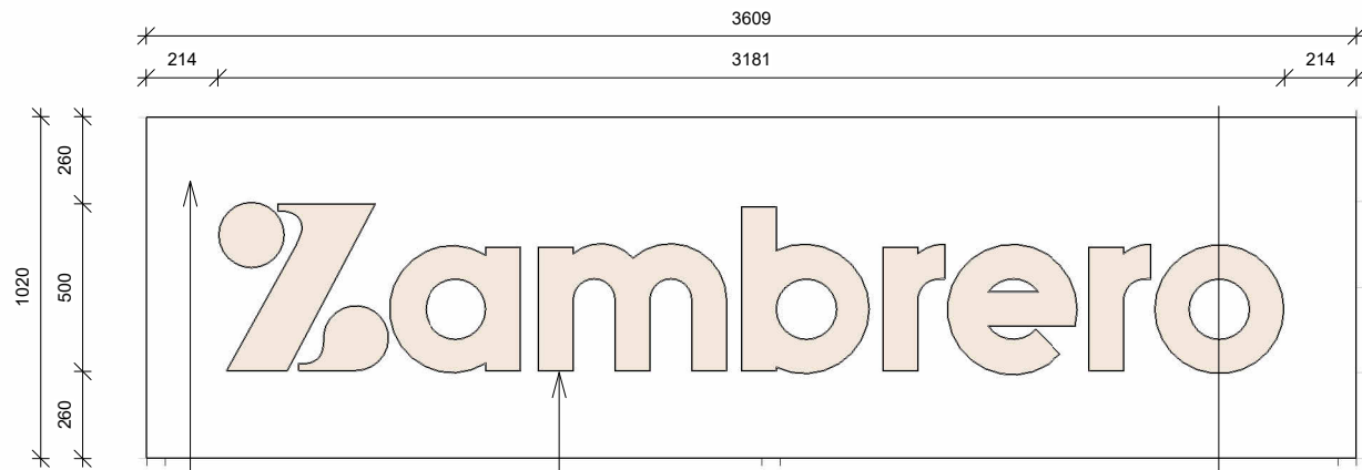
3 SIGN 01 D200 1 : 25
