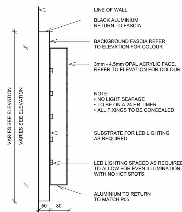
4 LIGHTBOX SECTION D200 1 : 10
