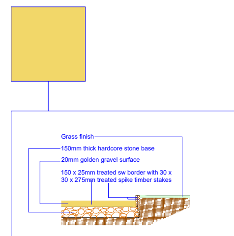
M5 - GRAVEL PATH & TIMBER BORDER
