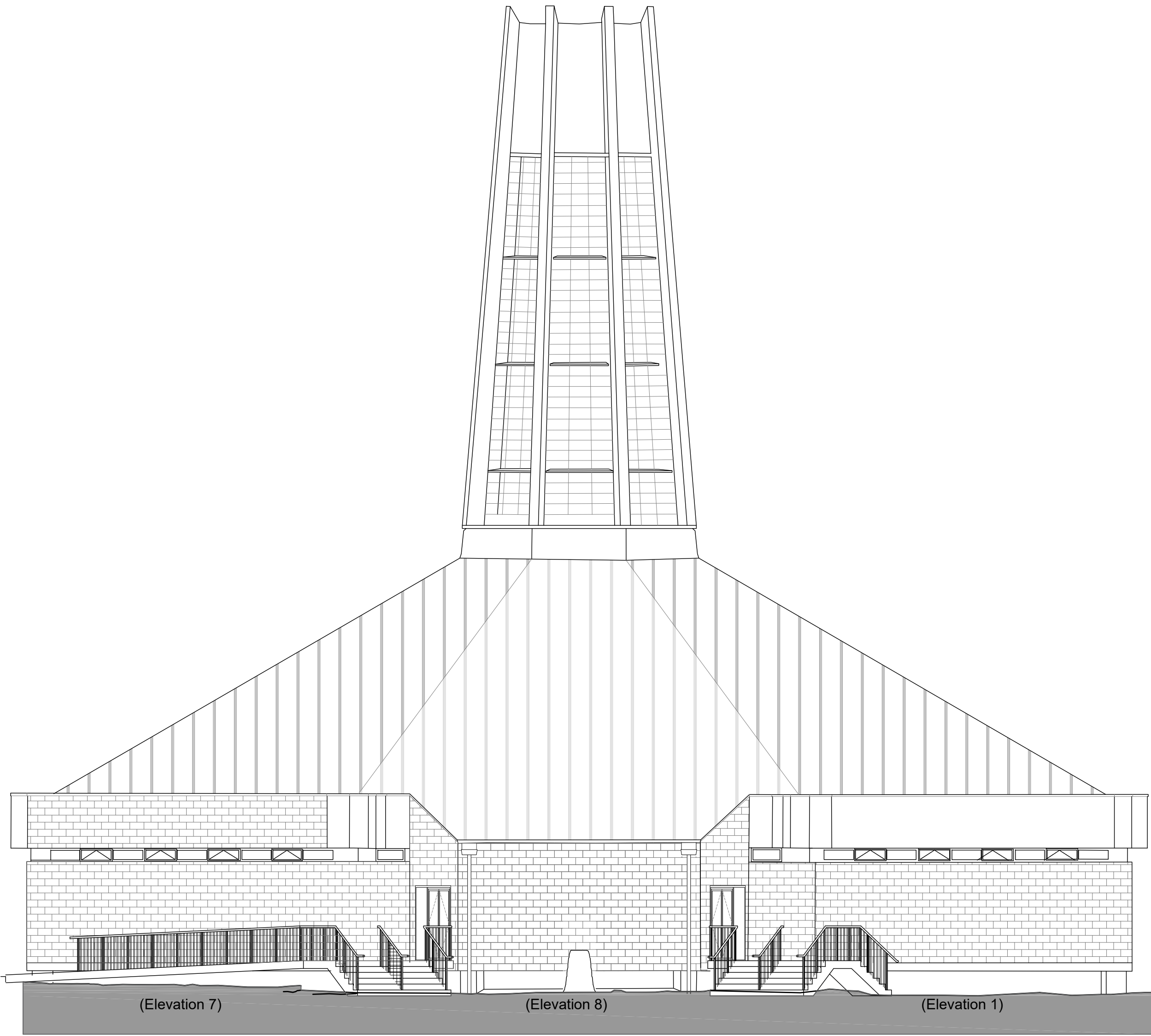
Elevation A
